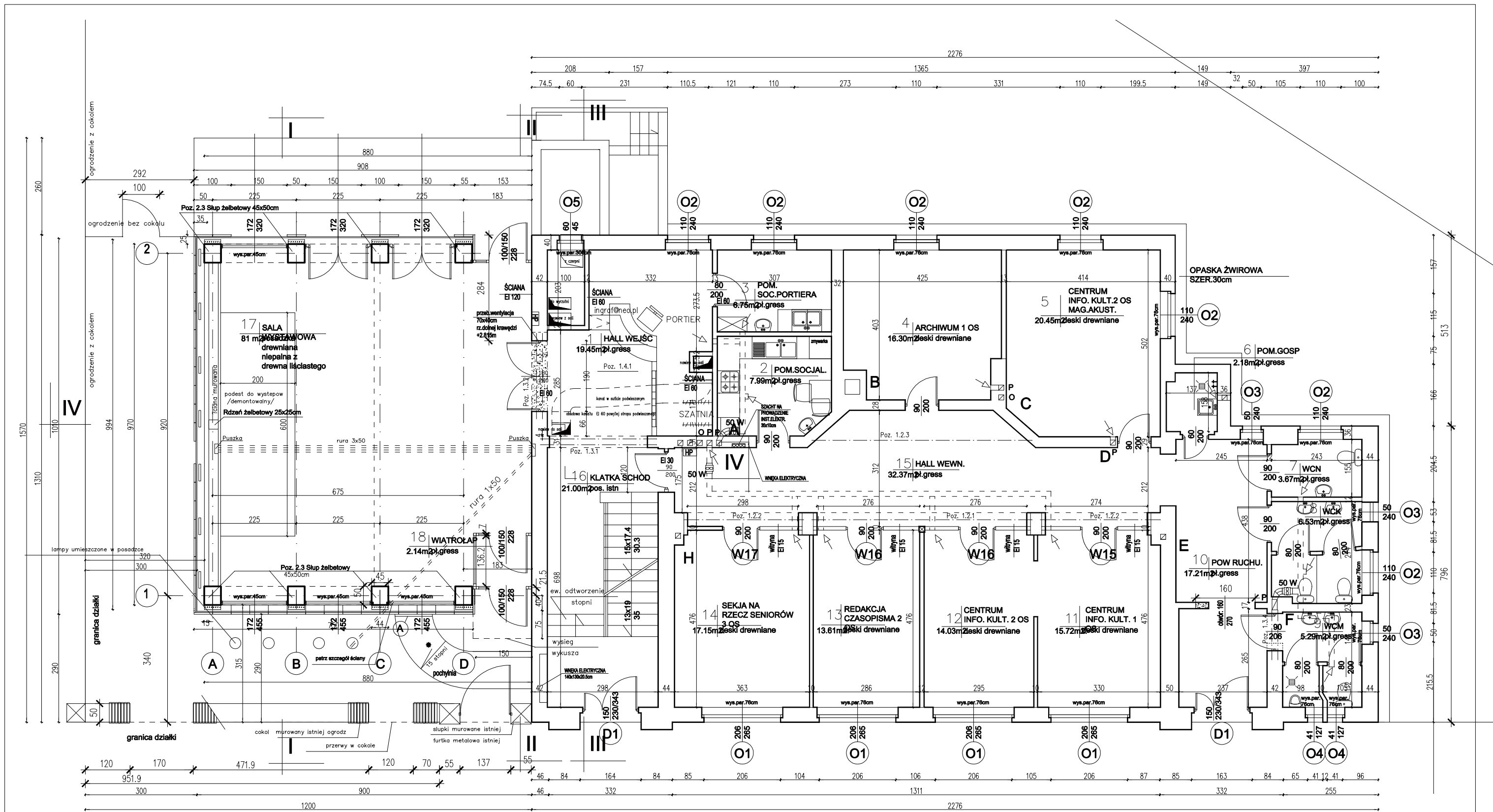
RZUT PARTERU 1:100
