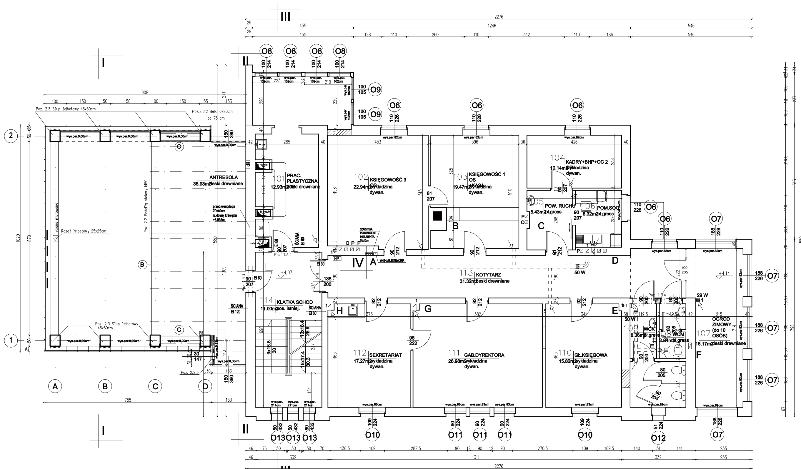
RZUT I PIĘTRA 1: 100
